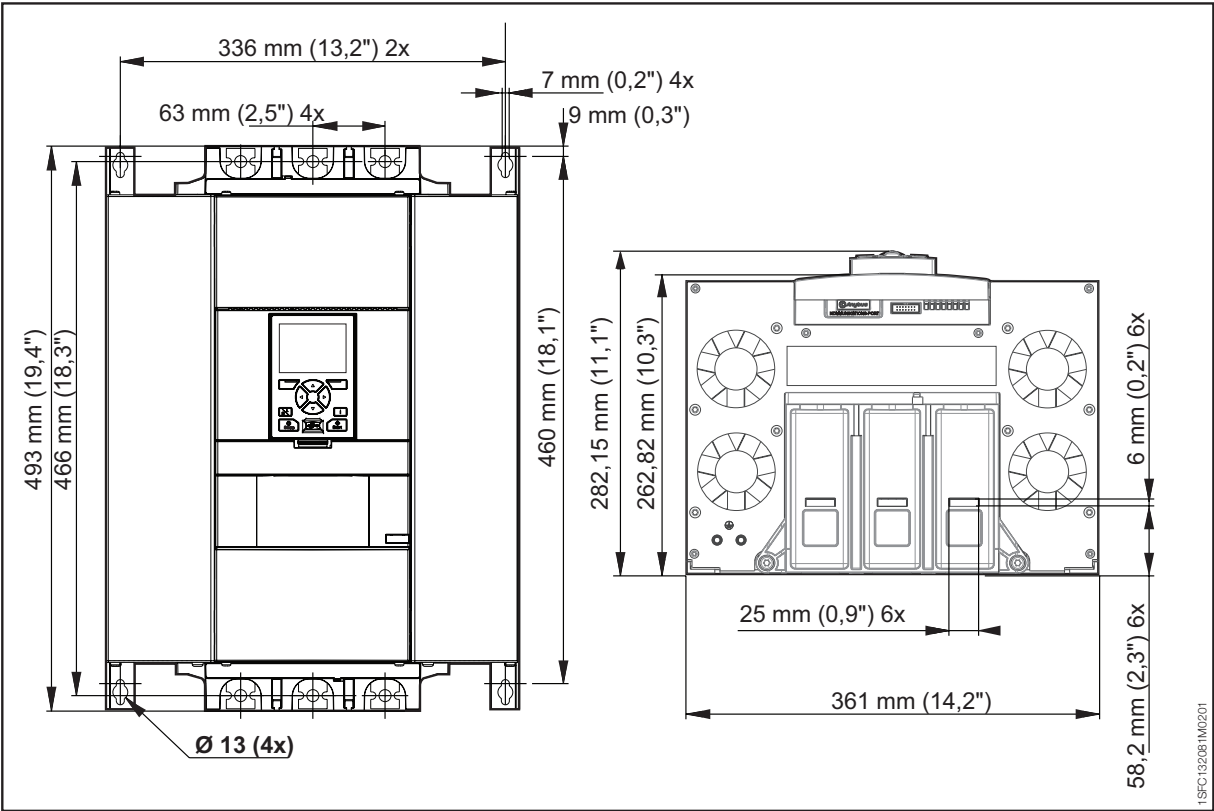
Abbildung 3.6 Abmessungen PSTX470..570
