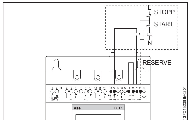
Abbildung 5.8 Konventionelle Schaltung (durchgehendes Startsignal erforderlich)
