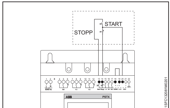
Abbildung 5.7 Warteschaltung (Puls für Start genügt)
