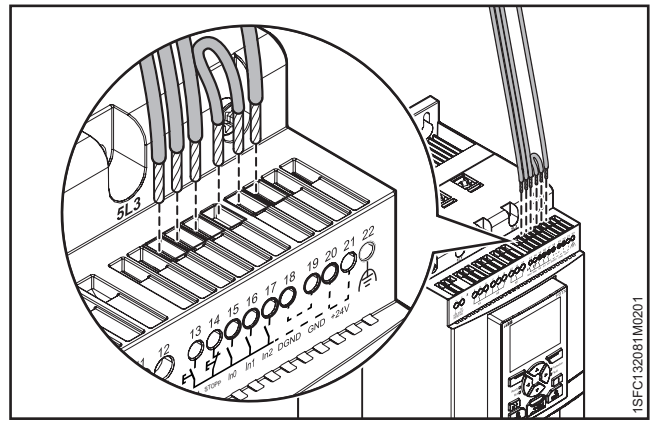
Abbildung 5.11 Klemmen 16 und 17
