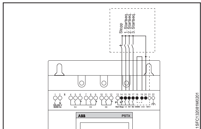
Abbildung 5.16 Interne Steuerspannung
