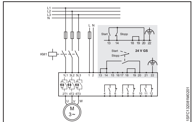
Abbildung 2.5 Schaltplan (Sicherungs- und Schützversion)
