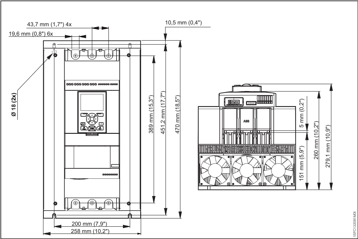
Abbildung 3.5 Abmessungen PSTX210..370
