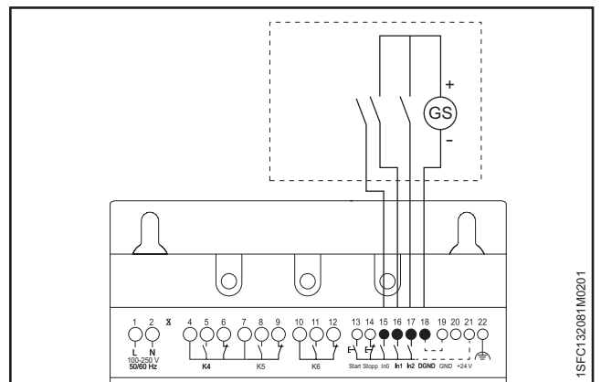
Abbildung 5.13 Externe Steuerspannung
