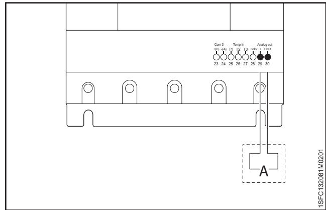
Abbildung 5.24 Analoger Ausgang
