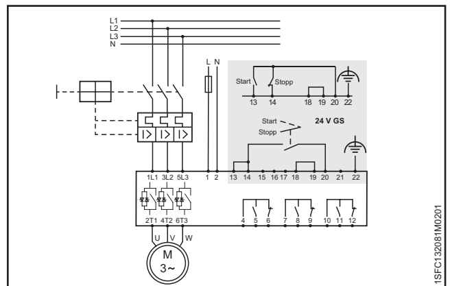
Abbildung 2.6 Schaltplan (MCCB-Version)
