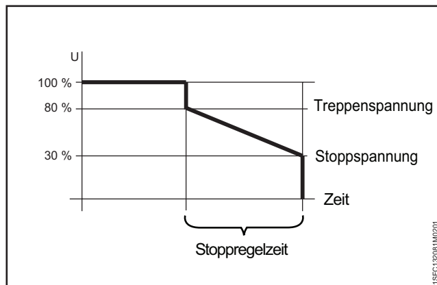
Abbildung 7.3 Spannungs-Stoppregelung
