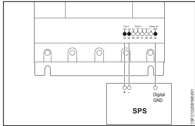
Abbildung 5.20 Modbus-RTU
