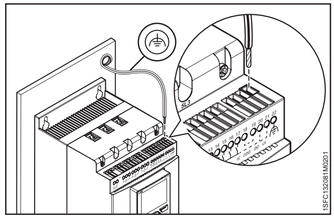
Abbildung 2.4 Funktionserde, Klemme 22
