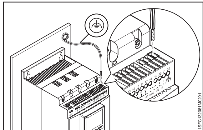
Abbildung 5.5 Funktionserde, Klemme 22
