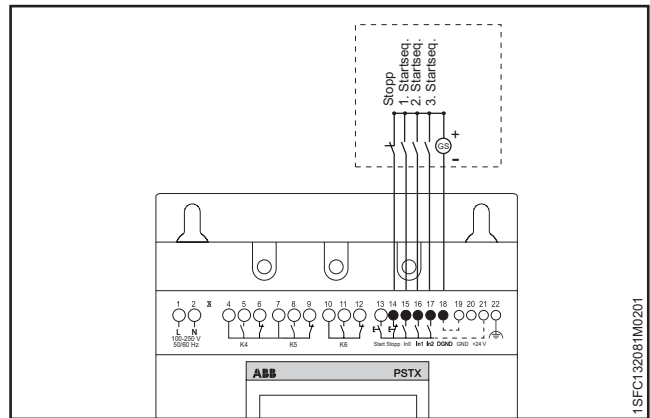
Abbildung 5.15 Externe Steuerspannung
