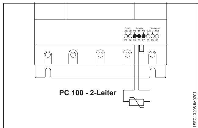
Abbildung 5.22 PT100 - 2-Leiter
