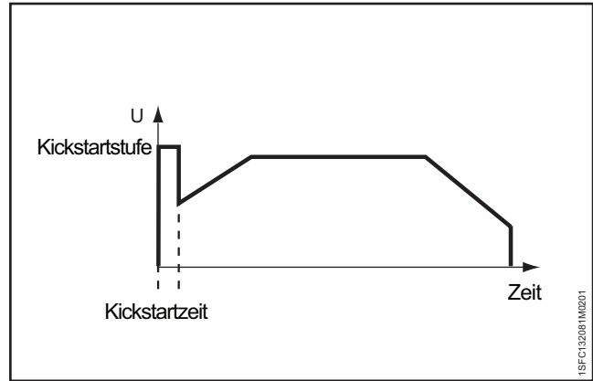
Abbildung 7.7 Kickstart
