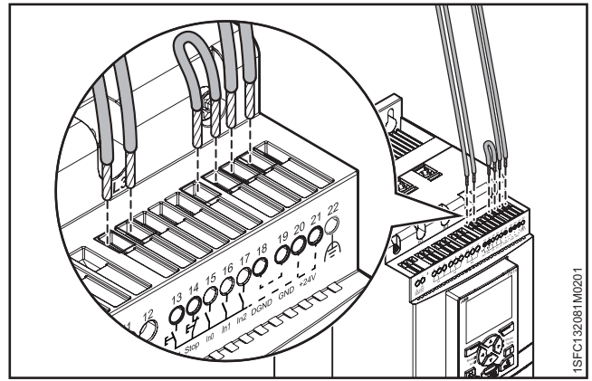
Abbildung 5.6 Start und Stopp, Klemmen 13, 14, 18, 19, 20, 21
