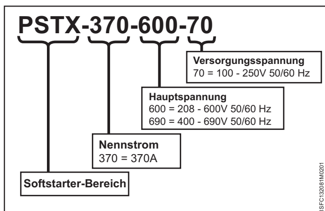
Abbildung 3.2 Typenbezeichnung
