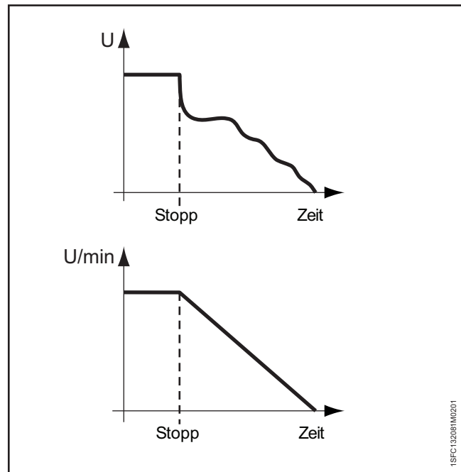
Abbildung 7.5 Drehmoment-Stoppregelung
