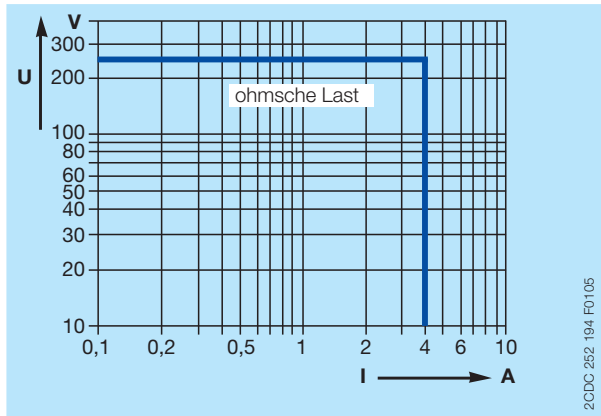
AC-Last (ohmsch)
