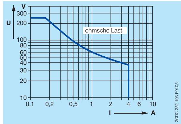
DC-Last (ohmsch)
