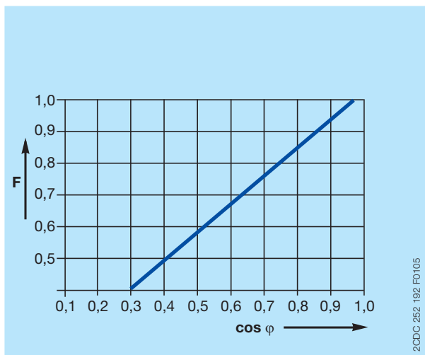
Reduktionsfaktor F bei induktiver AC-Last
