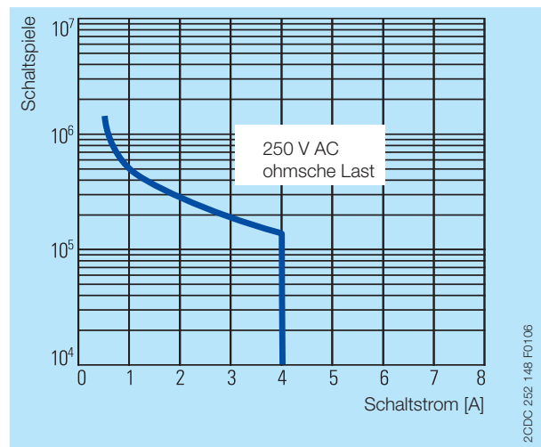
Kontaktlebensdauer / Anzahl der Operationen N 220 V 50 Hz 1 AC, 360 Operationen/h
