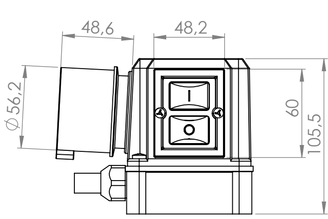
Ansicht "A"
