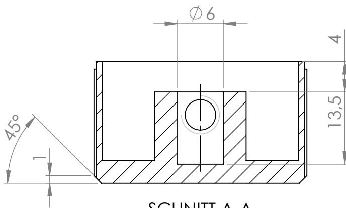
SCHNITT A-A
