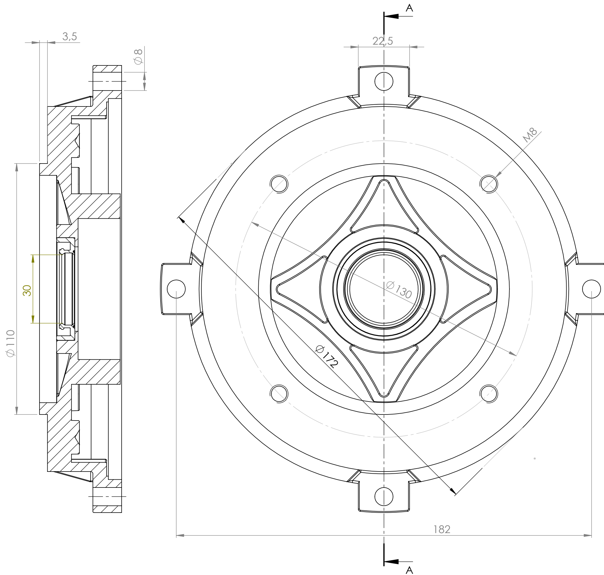
SCHNITT A-A
