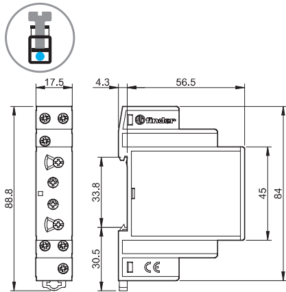
Typ 80.82 Schraubklemmen
