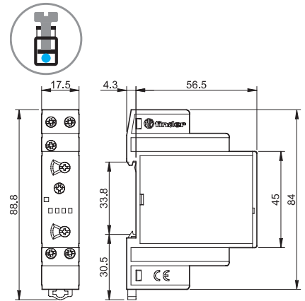
Typ 80.71 Schraubklemmen
