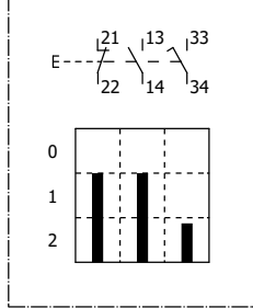
Schaltelement pro Taster
