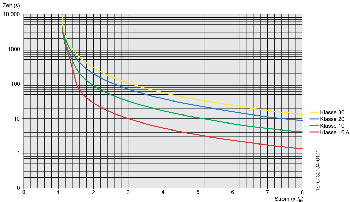
Auslösekurven des elektronischen Überlastschutzes (Kaltzustand) für PSTX und PSTB.
